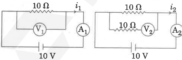
परिपथ 1
